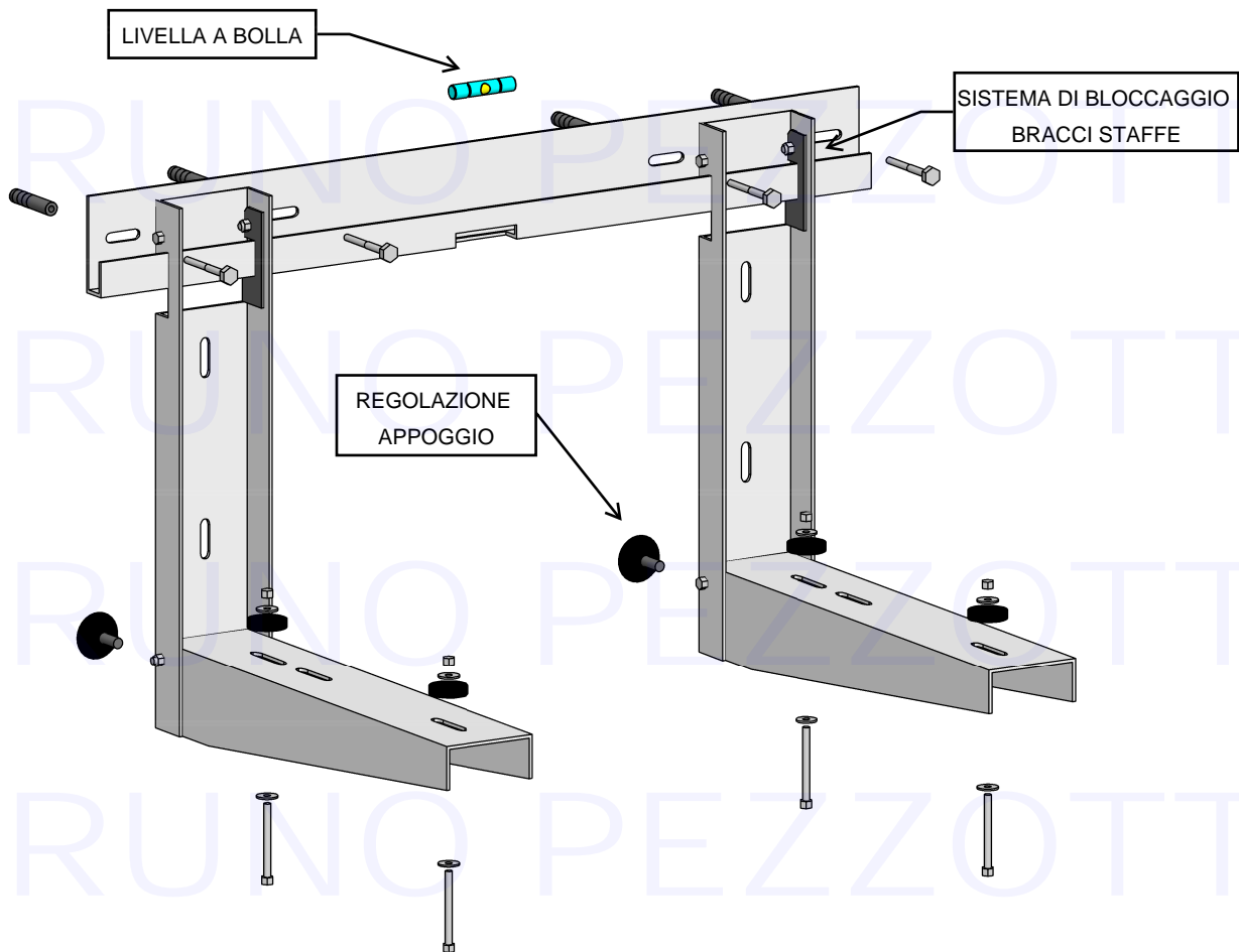
ASSONOMETRIA MONTAGGIO STAFFE AXONOMETRY MOUNTING BRACKETS
